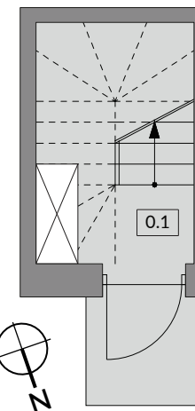
RZUT PARTERU
