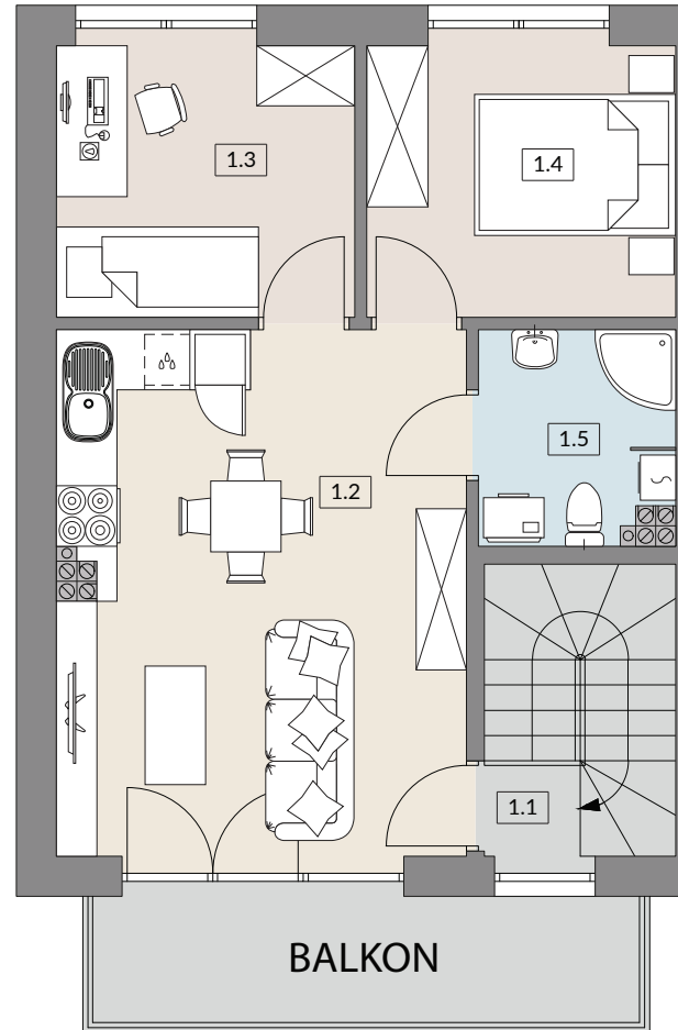
RZUT PIĘTRA
