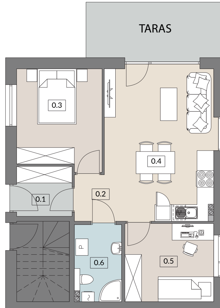
RZUT PARTERU
